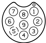
SOLDER LUG VIEW
